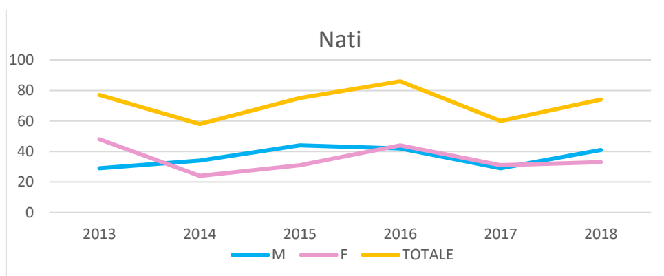
Grafico 1: Numero nati dall'anno 2013 all'anno 2018. Caerano di San Marco
